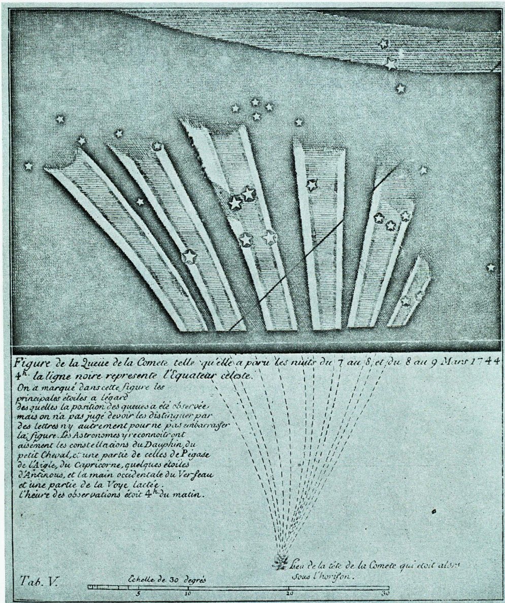
De grote komeet van 7-8 en 9 maart 1744. (Fig 46, Plaat XIII, uit het boek «The Story of the Comets» Getekend door De Chéseaux
