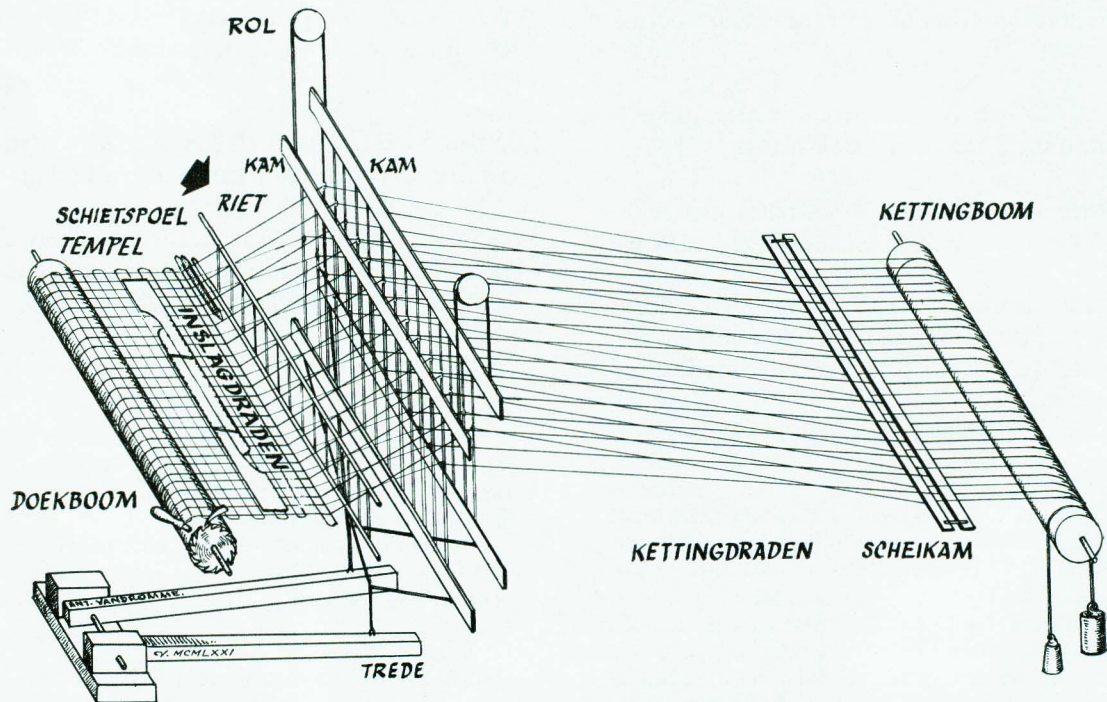
Weefgebouw met de diverse onderdelen. Letten we heel bijzonder op het RIET. J.B. Vandewalle was RIETMAKER van beroep.
