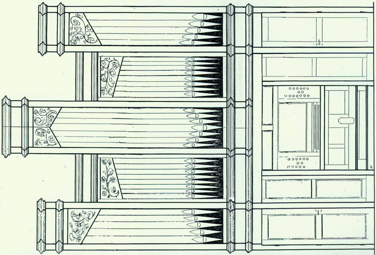
Ontwerptekening van het nieuwe orgel
