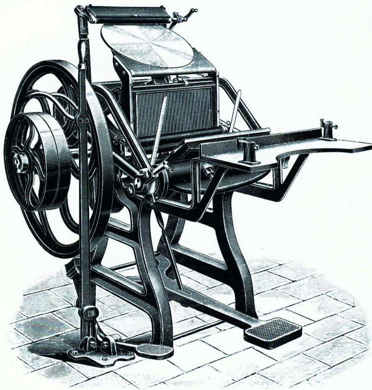
Trapdegelpers met tafelinktegeving "La Nationale" van Belgische makelij. Deze en vele andere degelpersen werden reeds vóór de eeuwwisseling tot ruimschoots na de tweede wereldoorlog intensief gebruikt in alle kleine drukkerijen.
