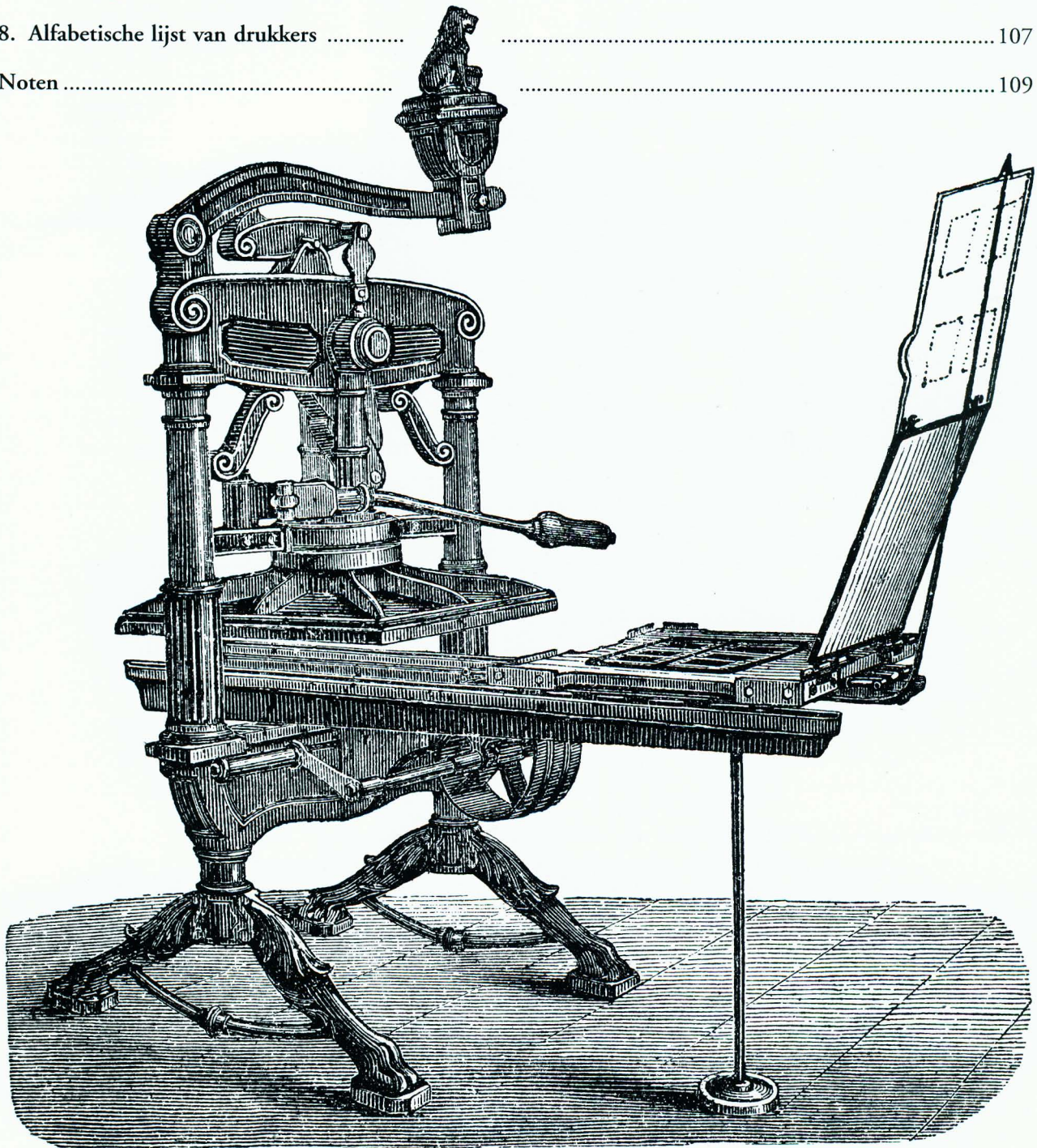
Handpers, voornamelijk gebruikt voor het drukken van notarisaffiches en pancartes, zoals er in België honderden hebben gewerkt tussen 1860 en 1960. Let op de Belgische leeuw op het tegengewicht, die verwijst naar de Belgische constructie van het geheel. (Doc. en repro Strobbe)
