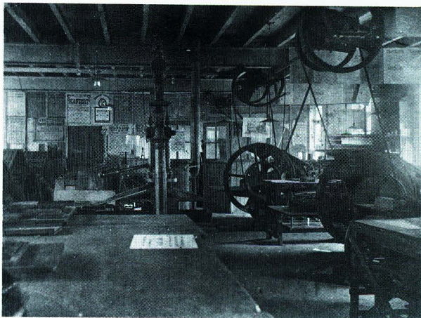
De werkplaats aan het Baertshof in een opname van juni 1918. Links de zetbokken, rechts twee cilinderpersen met aandrijfwerk en zijaanzicht van de Lejeune handpers met leeuw. Laatstgenoemde bevindt zich in het bedrijfsmuseum.
