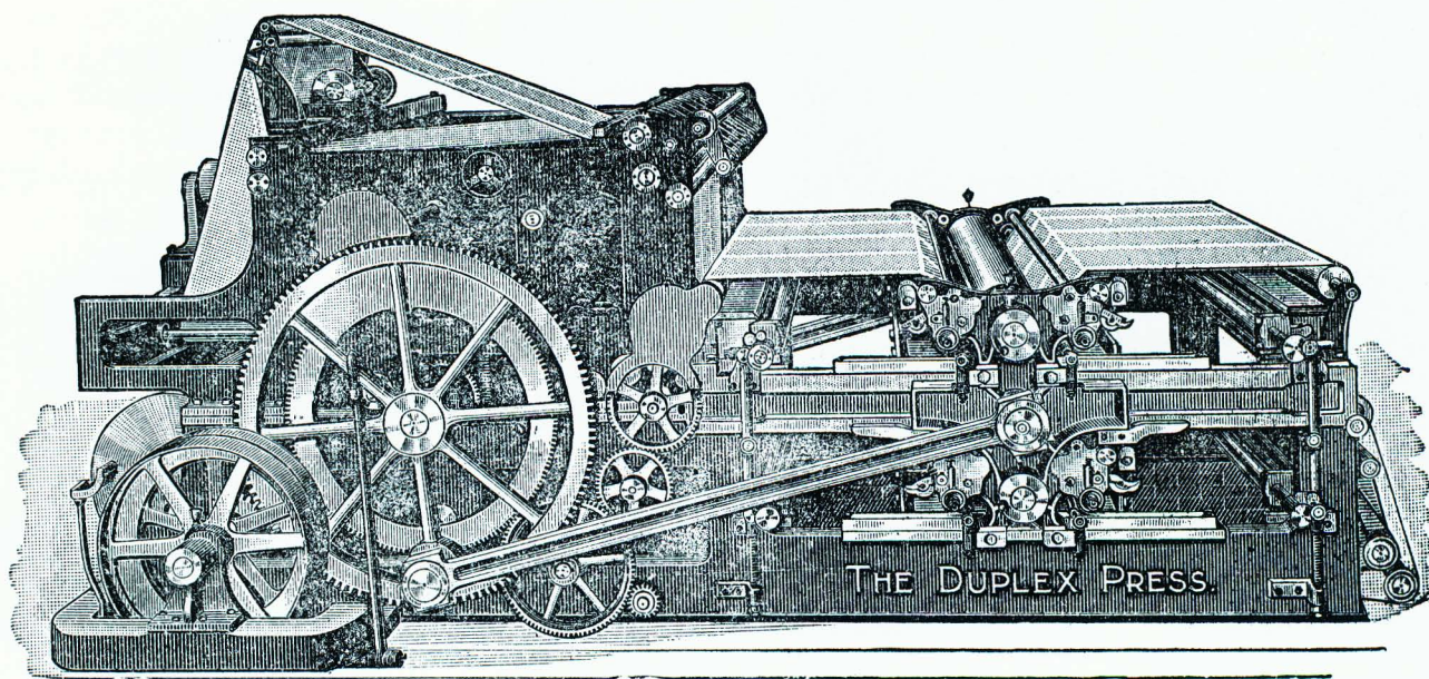
Reproductie van Strobbes "Sportvriend". Vanaf november 1910 werd deze krant gedrukt op een vlakke rotatiepers, de zogenaamde "Duplex Press". De drukvorm was vlak, het papier werd gevoed vanaf de bobijn en de gedrukte papierbaan werd automatisch gevouwen en gesneden aan 6000 exemplaren per uur (archief Drukkerij Strobbe).
